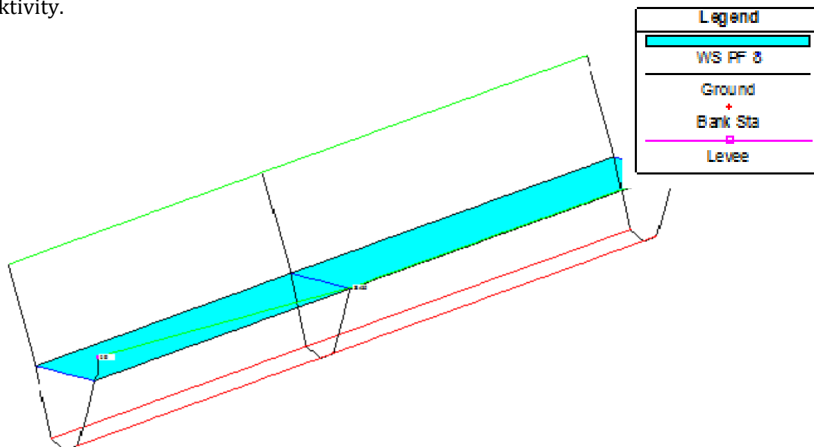
Charakteristika koryta při vybřežení
